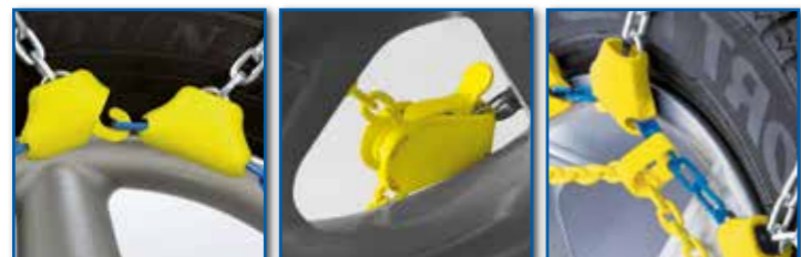
Durch thermoplastische Schutzelemente keine Berührungspunkte absence dans de zone de contact grâce aux éléments de protection thermoplastiques elementi di sicurezza termoplastici Kunststoffbeschichtetes Eisfrei Schnellverschluss-System système d'enclenchement rapide hors glace sistema rapido di chiusura placcato in plastica Abstandhalter bestimmen die Kettenführung des écarteurs de chaîne font office de guidage l'attacco a distanza determina la guida della catena
